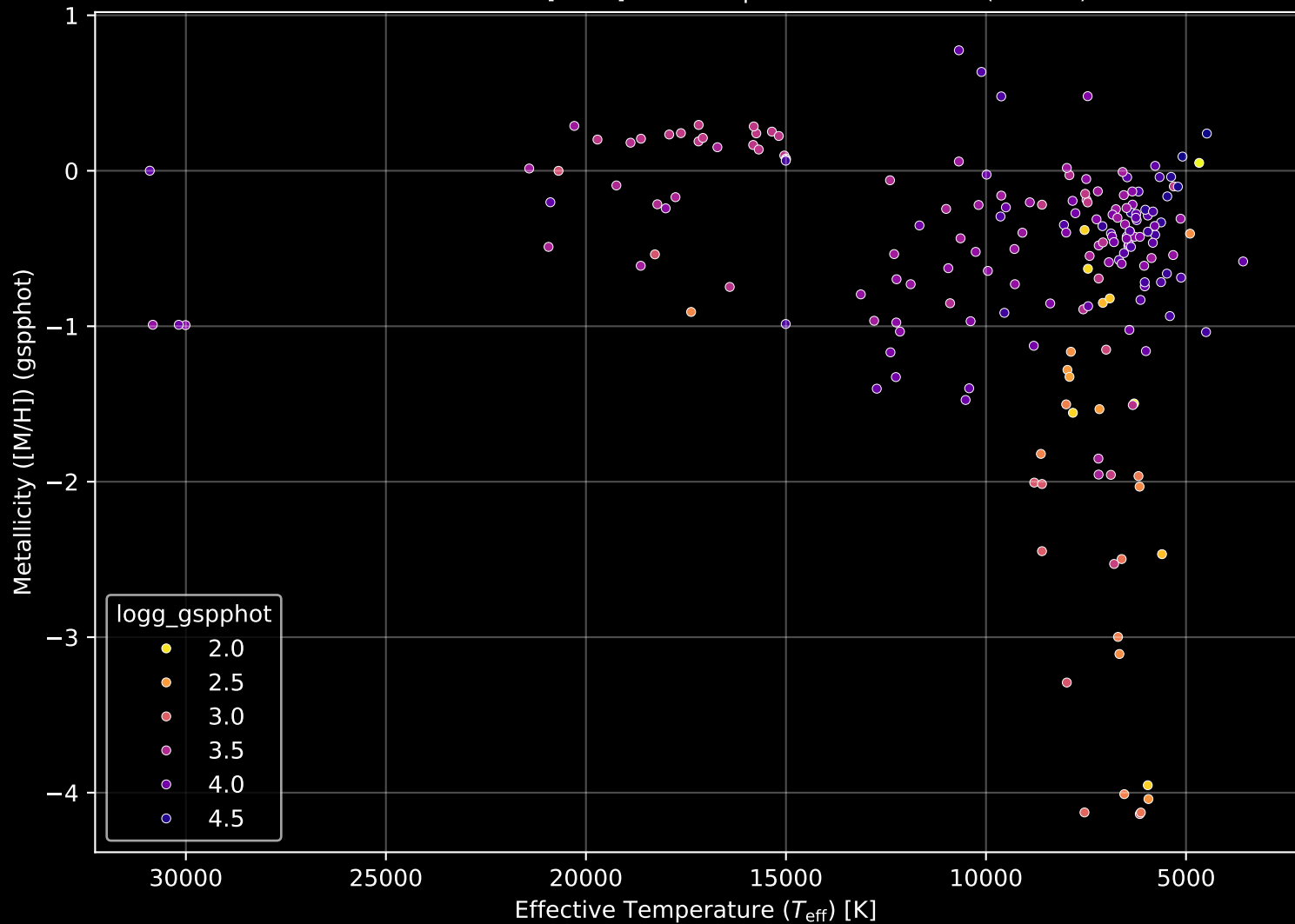
APOGEE DR17 Field: [W3-4] Stellar Population Parameters (n= 193)
